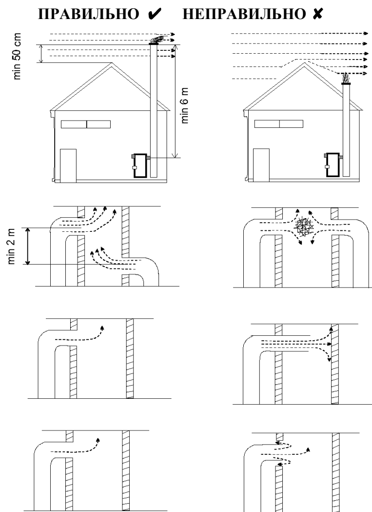
Рисунок 1. УСТАНОВКА ПЕЧИ
